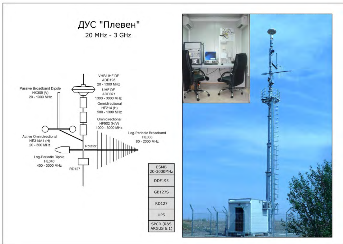
Фиг.2 - Общ вид на антенната мачта и контейнера.
