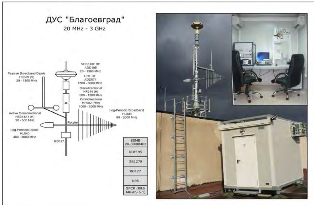
Фиг.1 - Общ вид на антенната мачта и контейнера.
