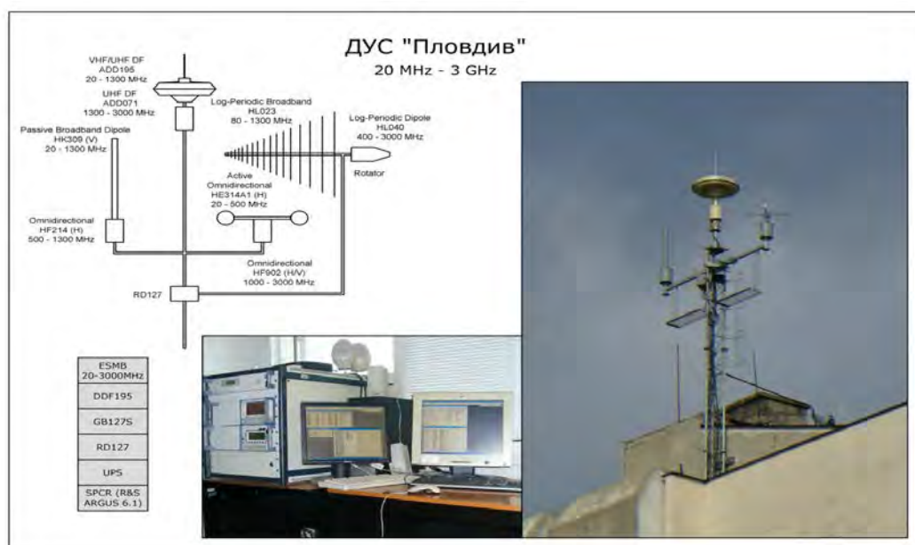
Фиг.3 - Общ вид на антенната мачта.
