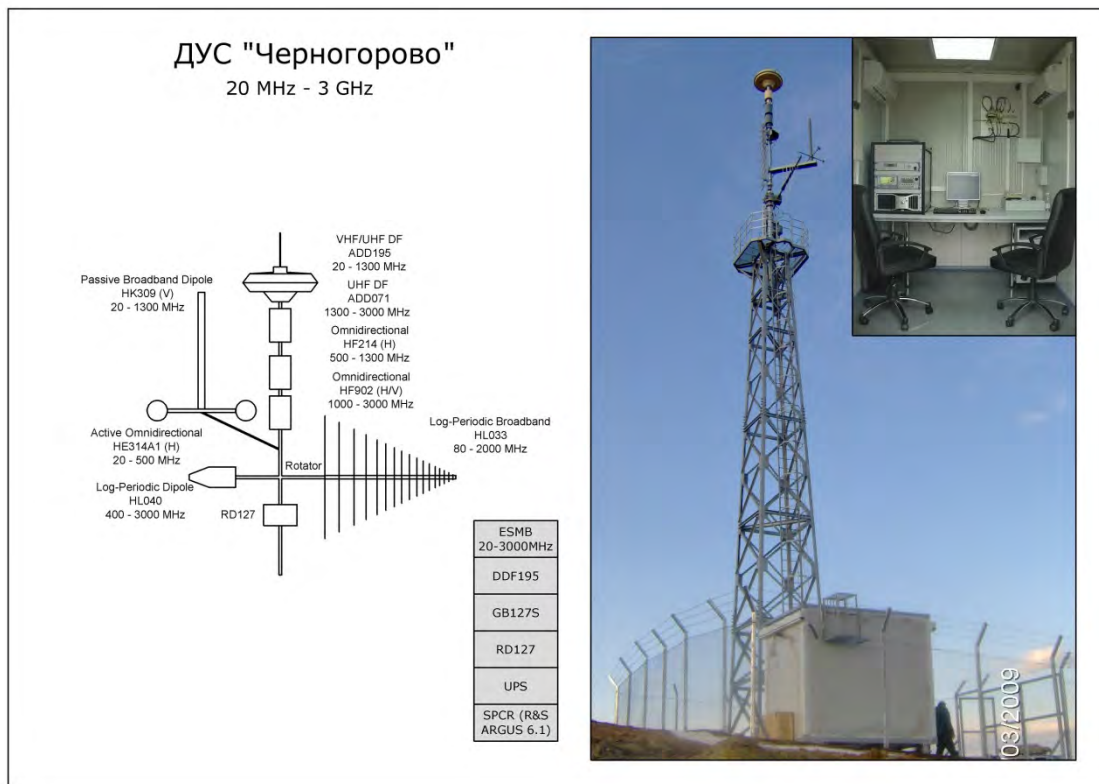
Фиг. 4 - Общ вид на антенната мачта и контейнера.
