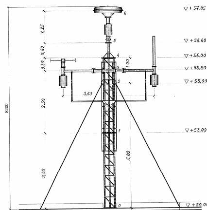
Антенен носач H = 8,0м
